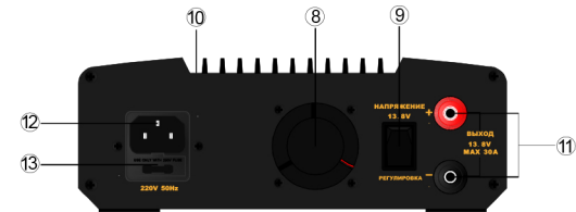
Вид сзади
